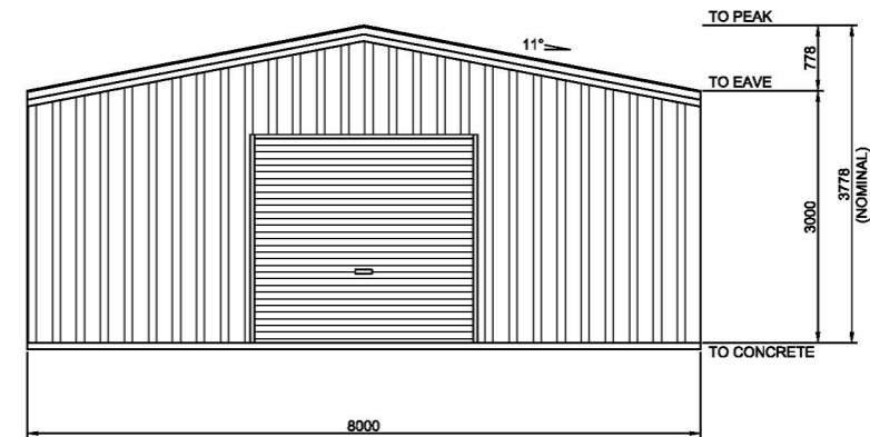
3 6 ENDWALL EXTERIOR ELEVATION SCALE: 1 = 100
