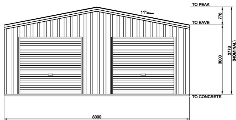
4 6 ENDWALL EXTERIOR ELEVATION SCALE: 1 = 100
